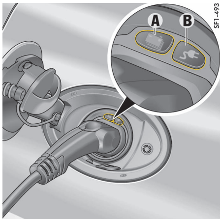
A 高压蓄电池充电状态 B 车辆插头连接状态
