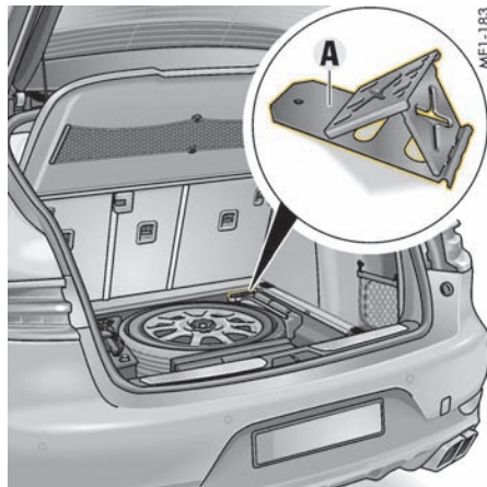
折叠车轮楔
