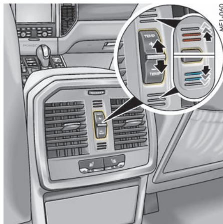
后部控制面板上的温度和风量控制装置（3区域空调系统）
