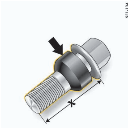
长车轮螺栓
