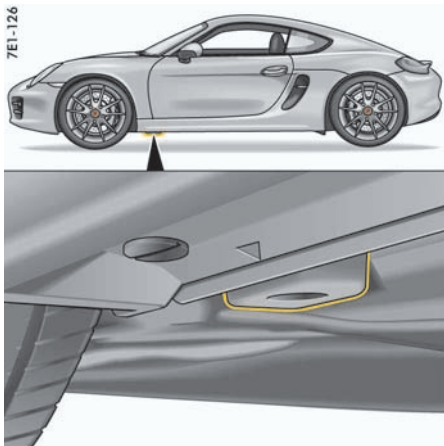
用于举升平台和千斤顶的前部举升点
