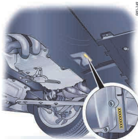
发动机号 在拆下车身底部护板后，可以看到压印在曲轴箱下侧的发动机号。
