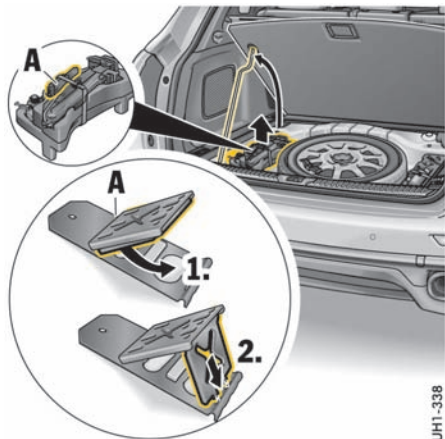
A · 车轮挡块
