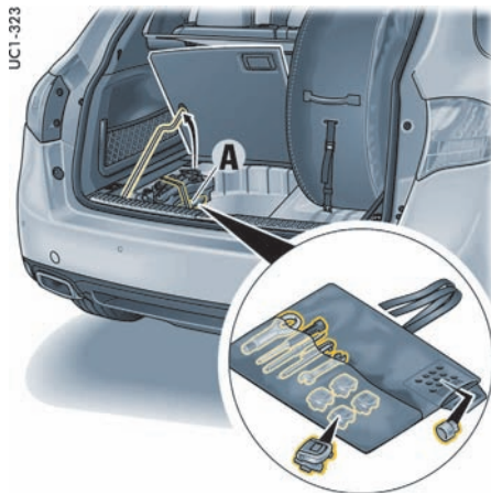
配备备用轮胎的车辆
