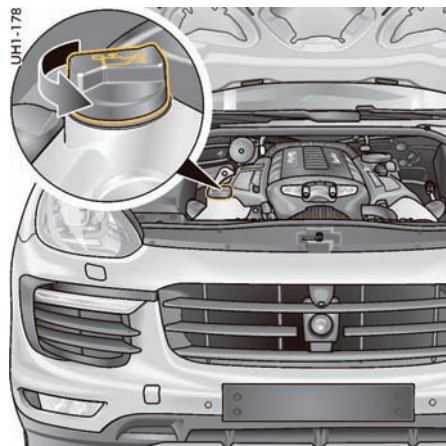
Cayenne Turbo、Cayenne Turbo S 上的机油加注点
