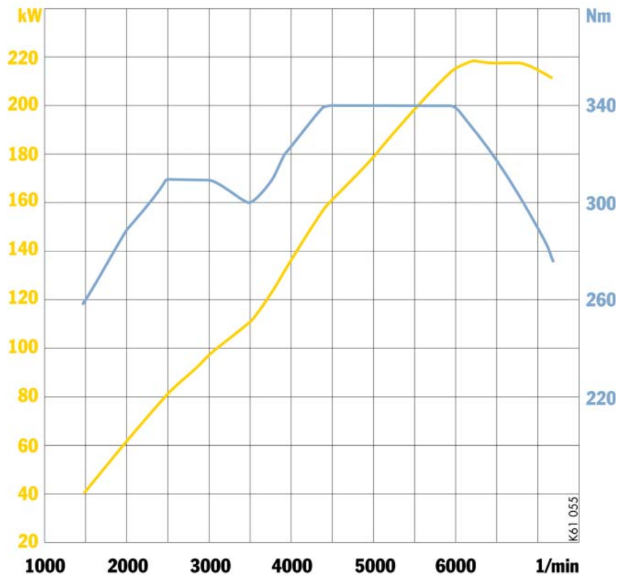
Boxster S: 全负荷的发动机曲线图
