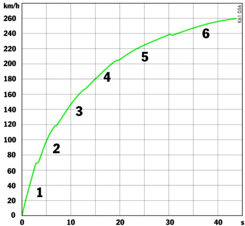
Boxster S: 加速特性曲线图
