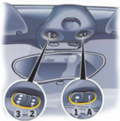
1、2、3 - 可编程按钮 A - 用于识别状态的发光二极管
