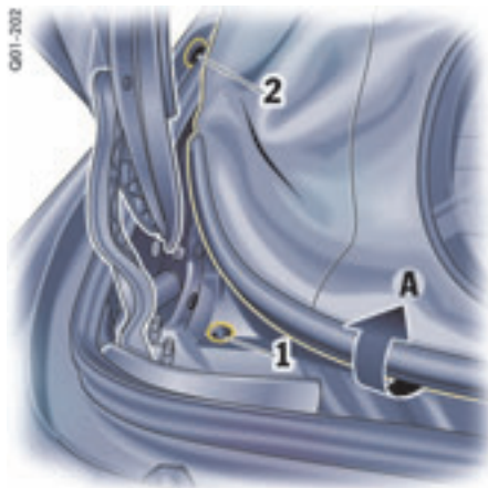
排水 (Boxster、Boxster S)
