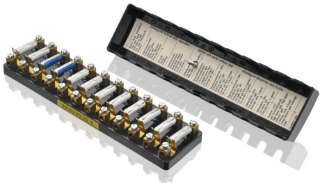
Scatola fusibili da 12 Codice 90161280120 Modello 911 F (1965–1968)
