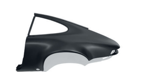
Pannello laterale in lamiera sottile, lato sinistro Codice 91150304501GRV Modello 911 F (1972–1973), solo per RS 2.7
